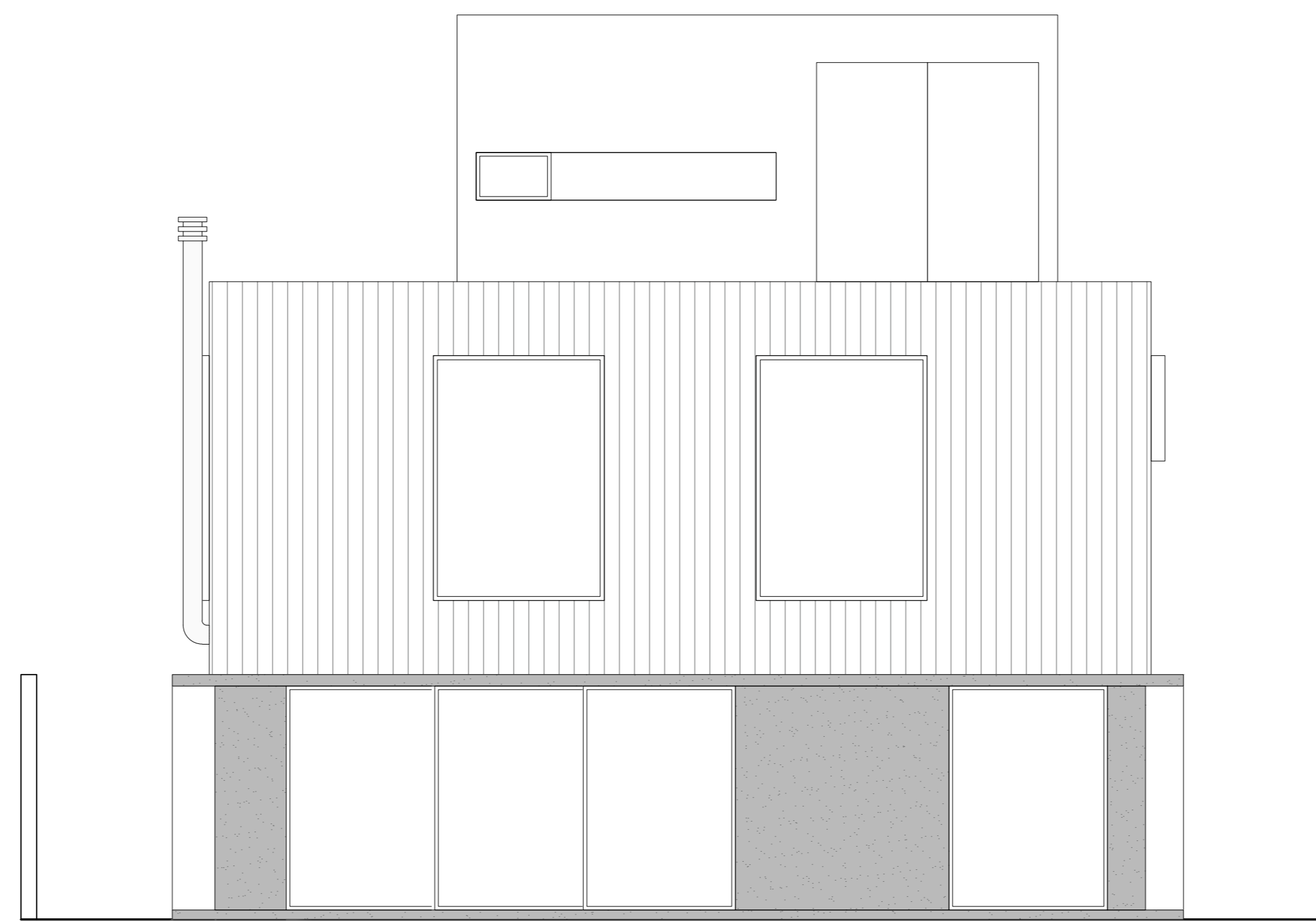
ELEVAÇÃO 2
