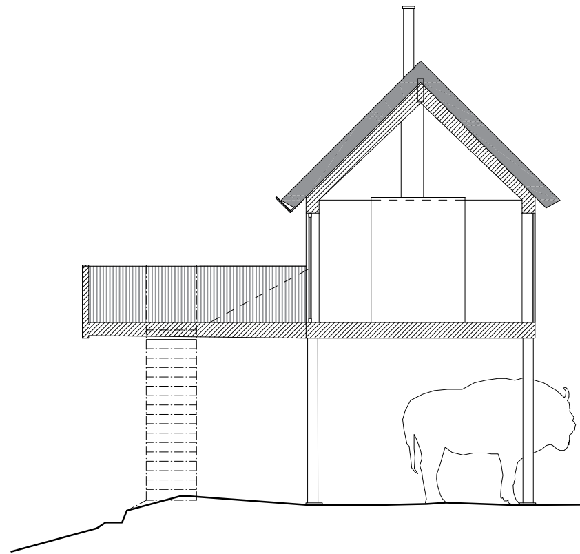
SEKTION A-A
