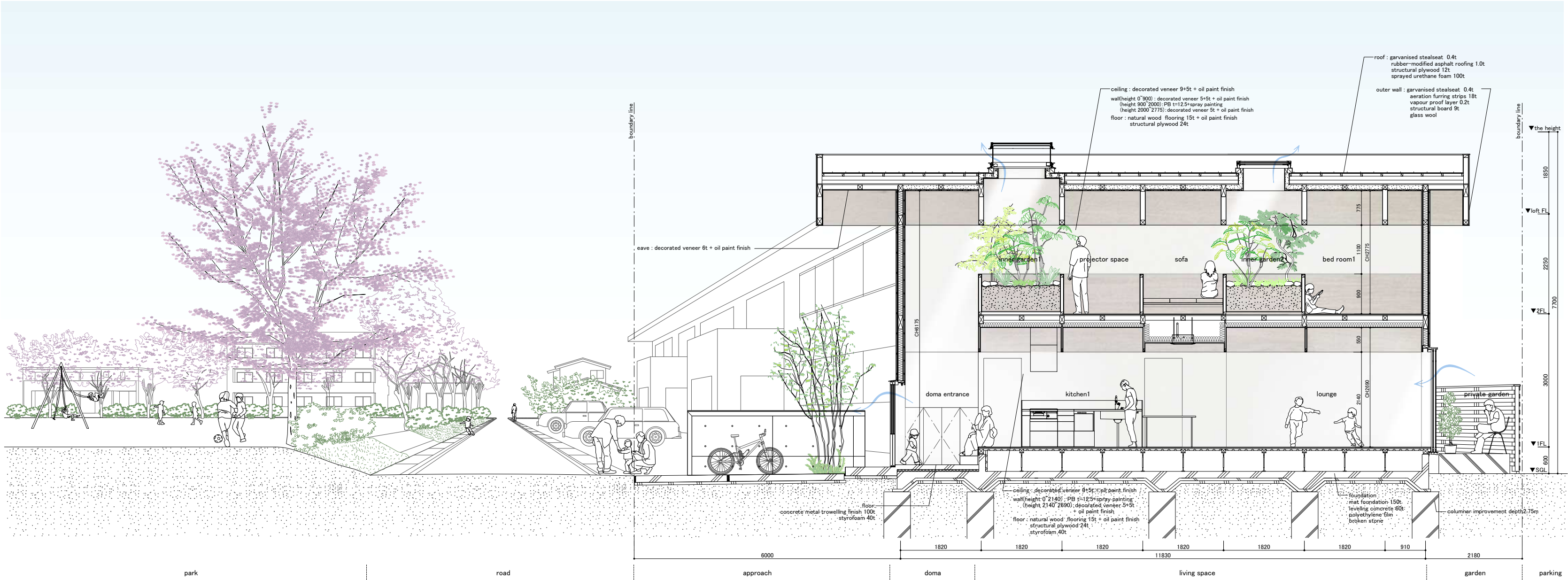
A-A' SECTION 1:80
