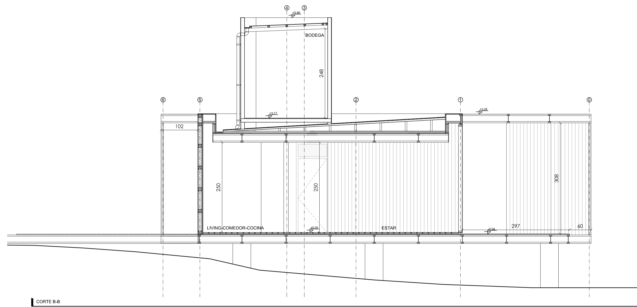
CORTE B-B
