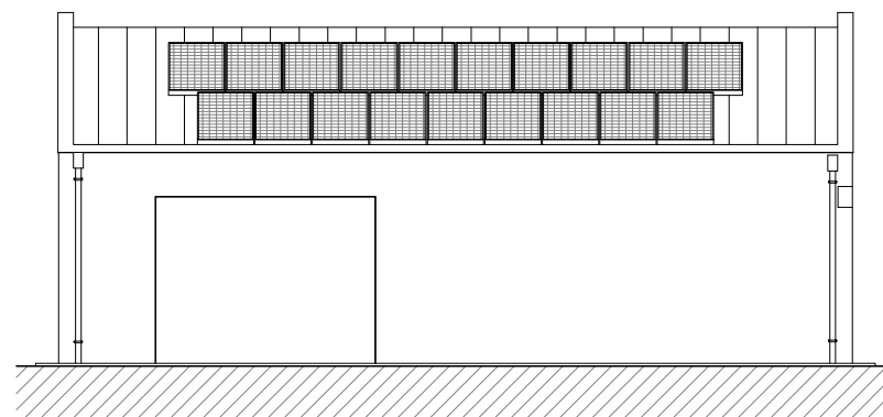
PROSPETTO SUD
