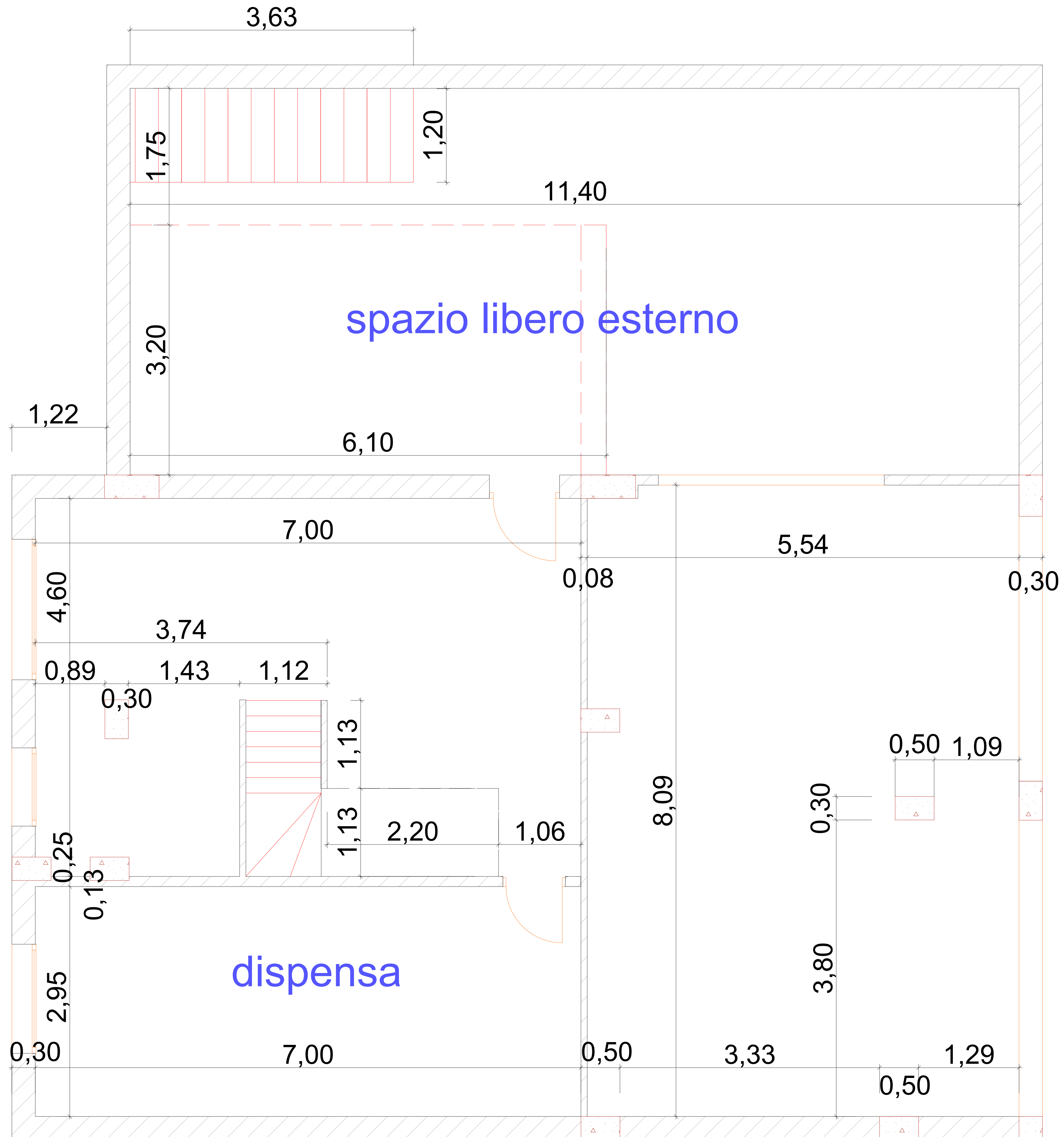
Pianta allo stato Passato Scala 1:25
