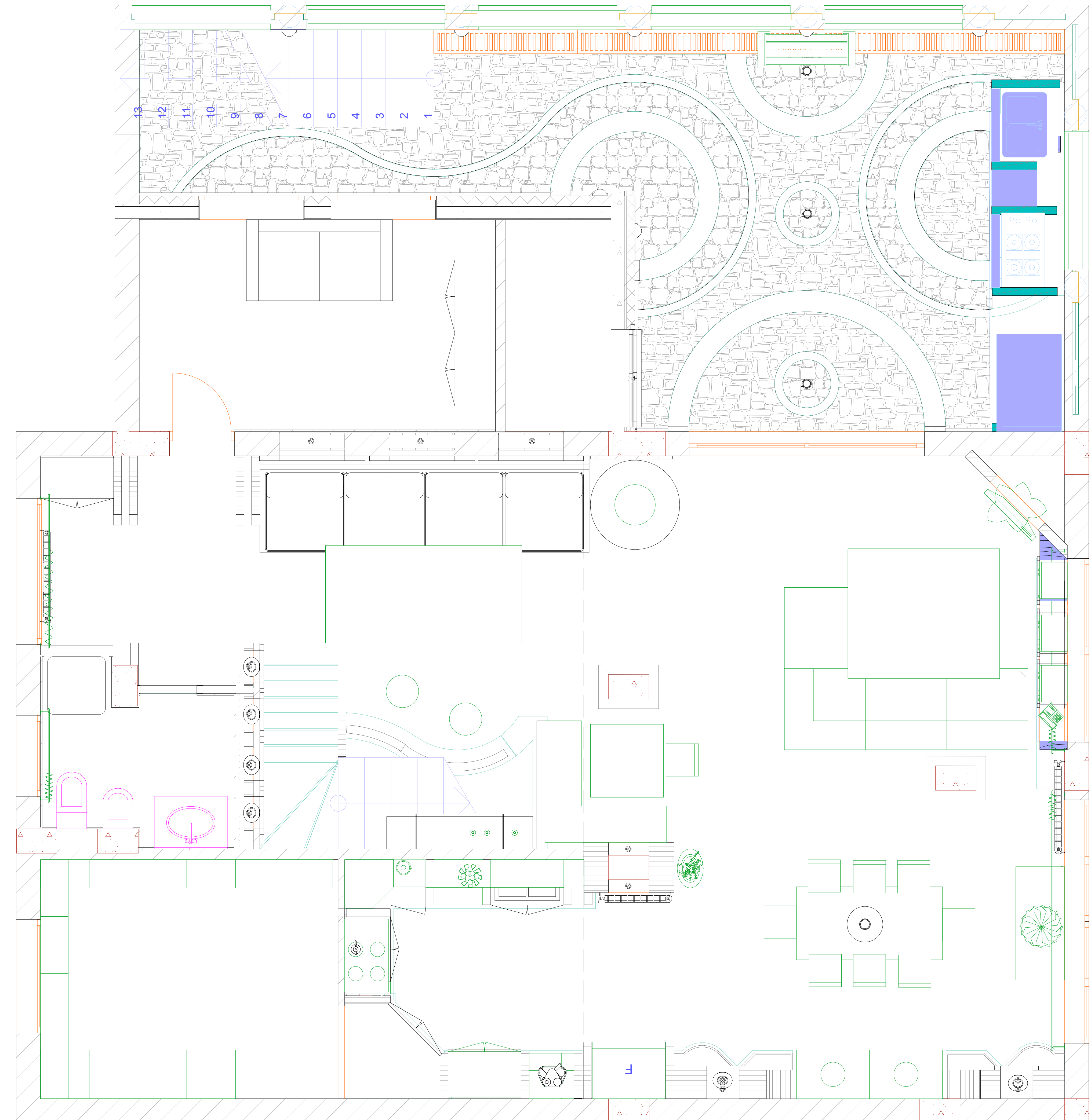
Pianta Ultimata rapp. 1:25
