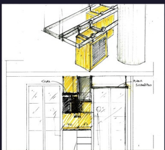
ESTUDIO DE LA ESTRUCTURA EN HIERRO
