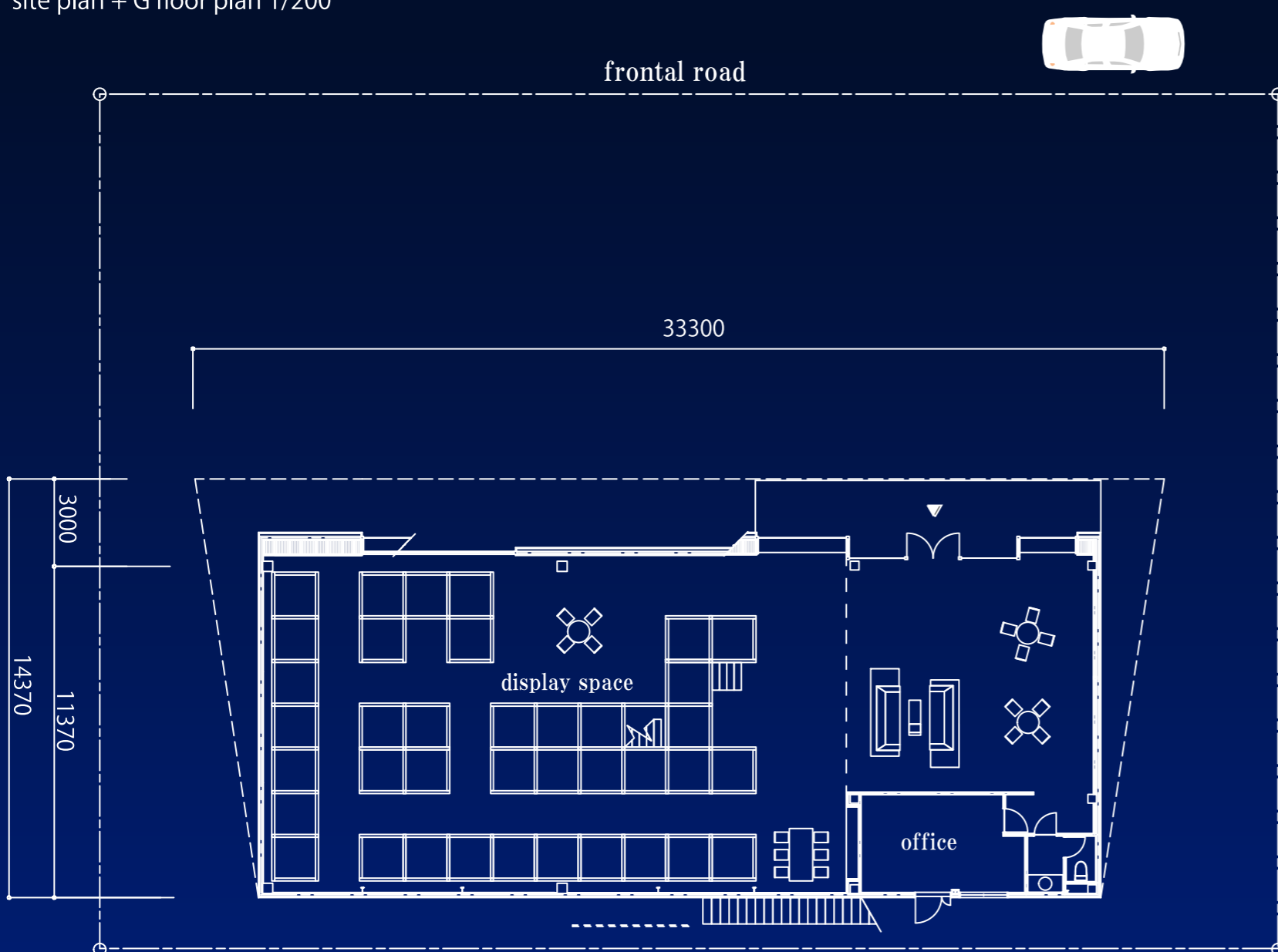
site plan + G floor plan 1/200
