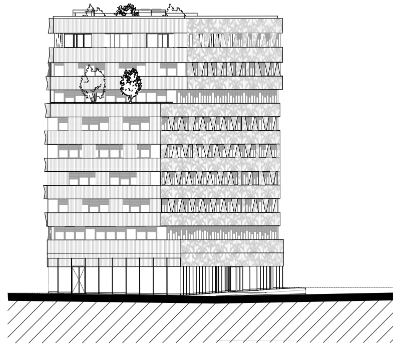
Coupe Sud-Est
