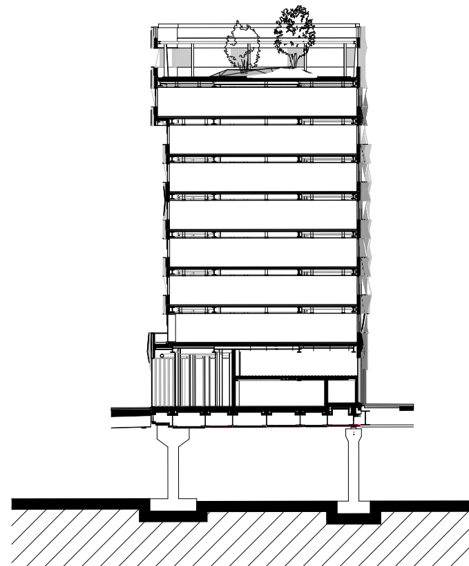
Coupe CC
