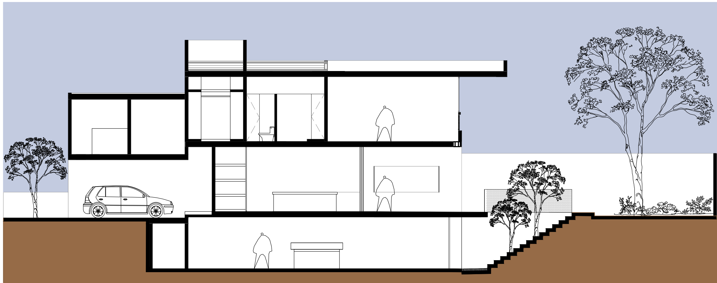
SECTION A-A'
