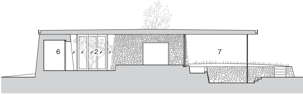
A-A' section
