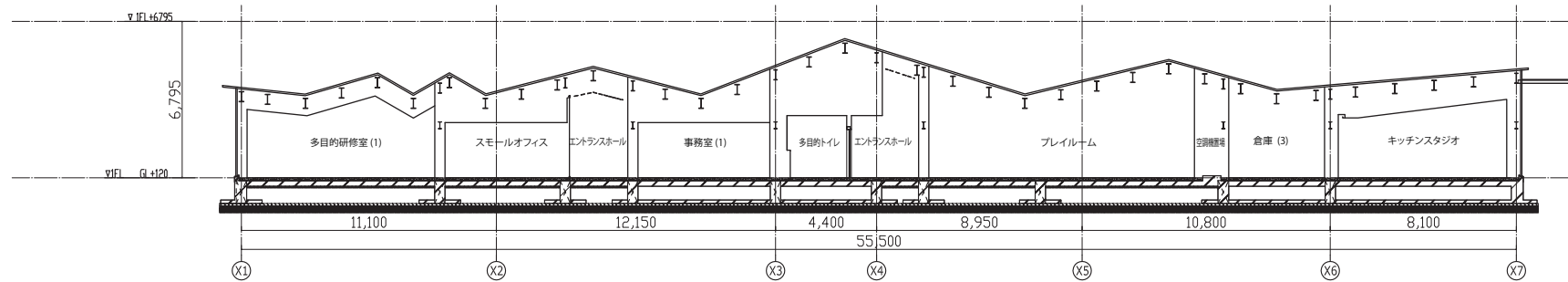
BB'断面図 1:300
